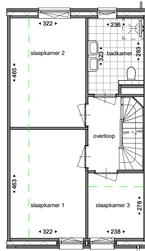
eerste verdieping
