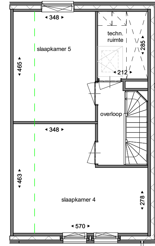
tweede verdieping
